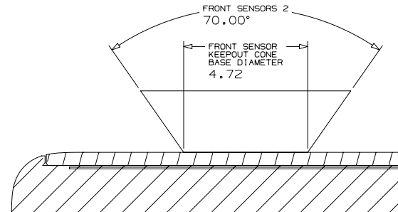
SECTION W - W
